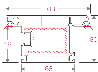
60IROSDS 60 Out Swing Door Sash
