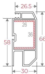
IRMS66 Mesh Door Sash 66
