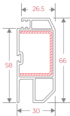
IRMS66 Mesh Door Sash 66
